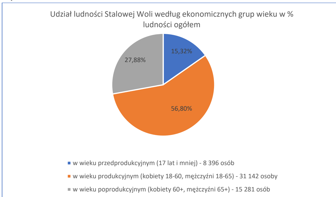
Wykres nr 3
